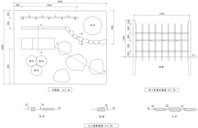
造園職種施工図(単位:mm)
