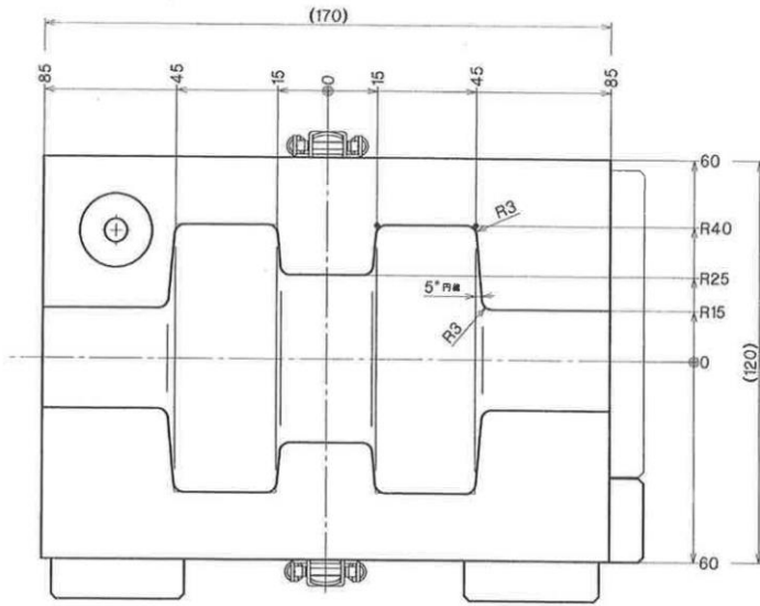
断面あ-あ
