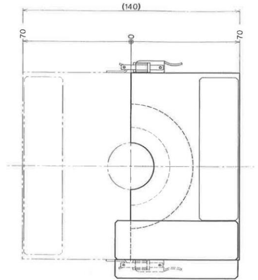
矢視 い
