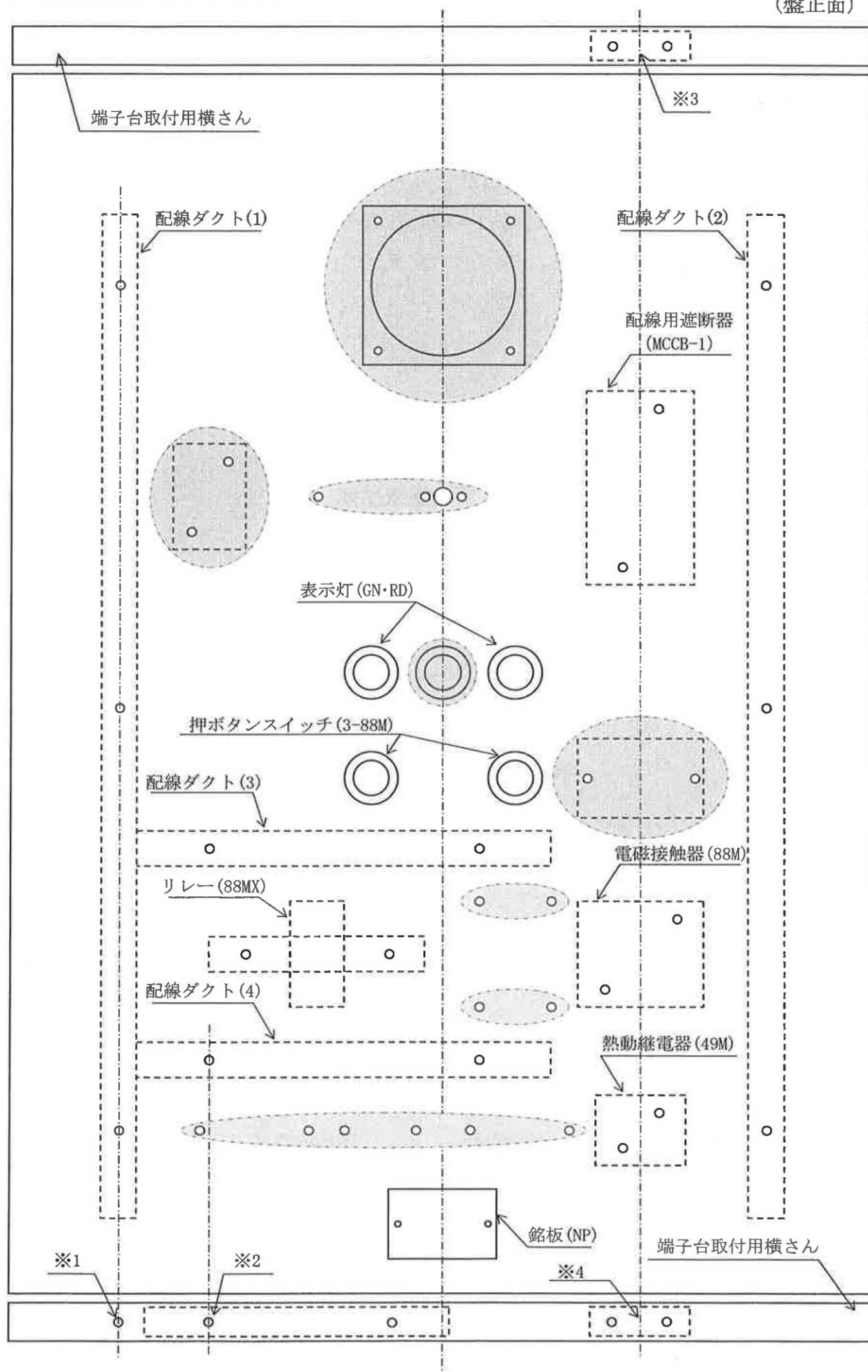
ロ. 盤面器具取付け穴位置配置図
