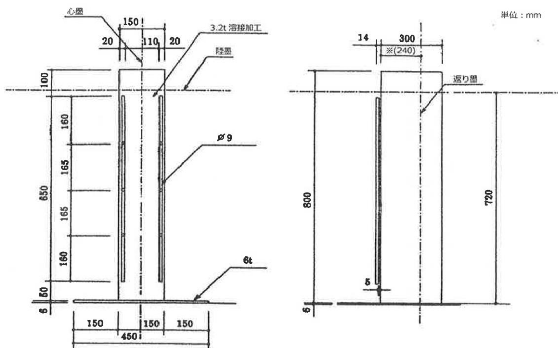
立面图
