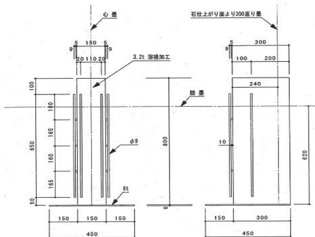
立 面 図
