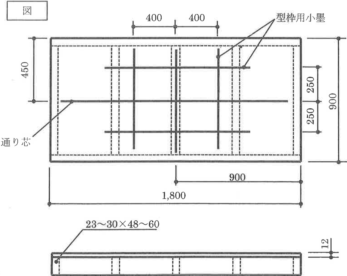
【基礎級】型枠施工(型枠工事作業) 型おこし台作成図 (単位:mm)
