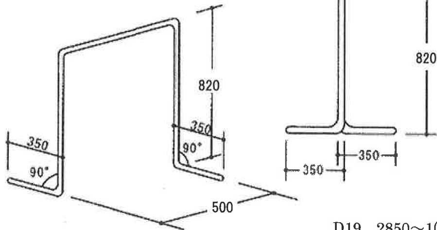
柱組立て用うま
