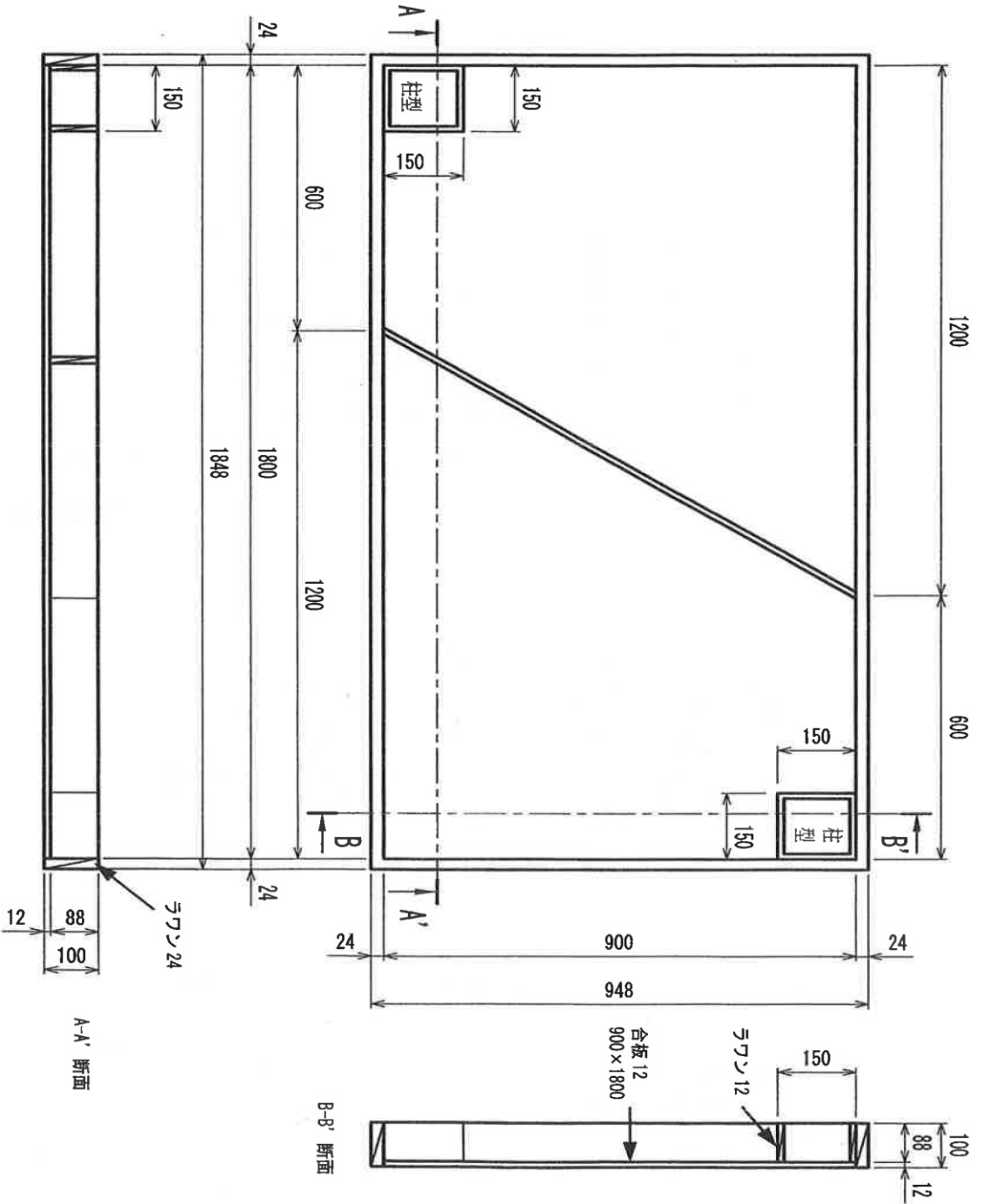
随時3級 内装仕上げ施工（プラスチック系床仕上げ工事作業）実技試験台製作図
