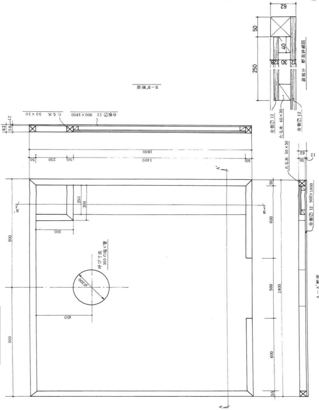
別添 随時2級 試験台製作図
