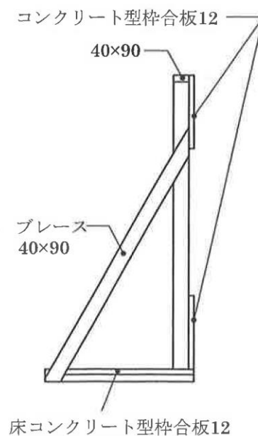
側面図
