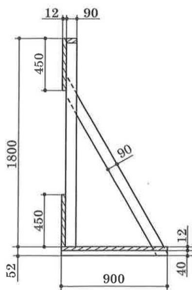
A-A'断面図
