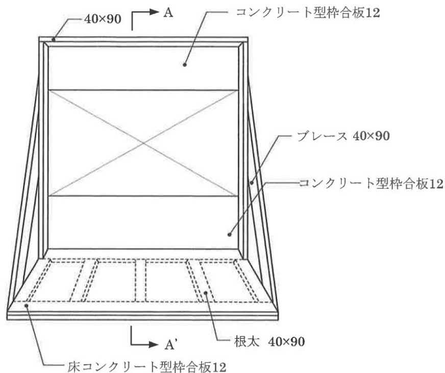
見取図
