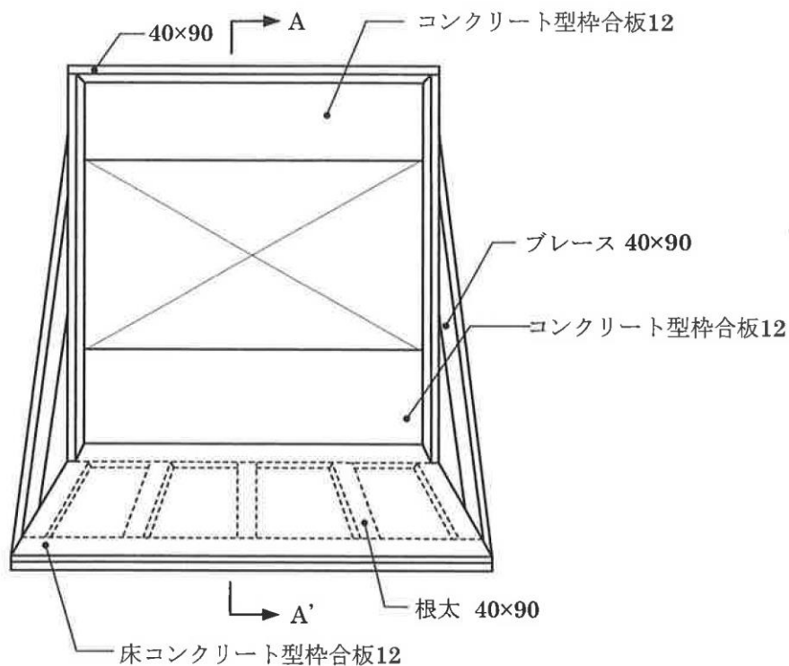
見 取 図
