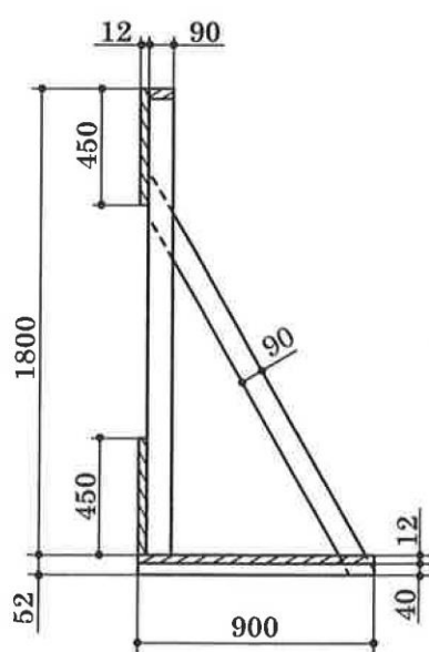
A-A' 断面図
