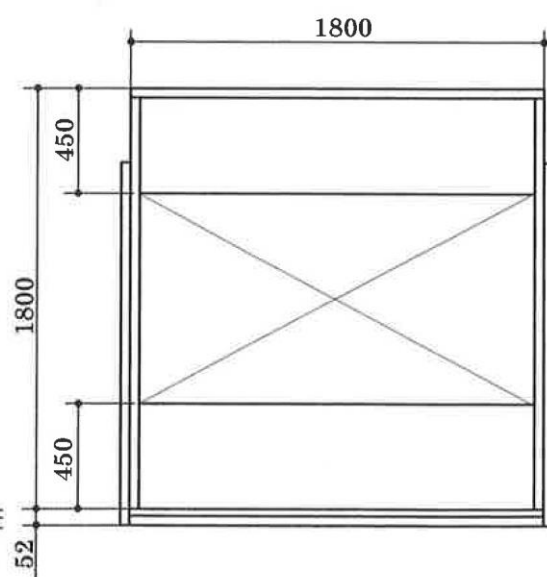
正面図
