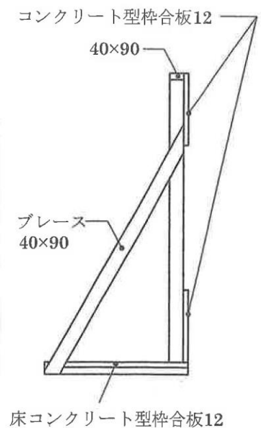
側 面 図
