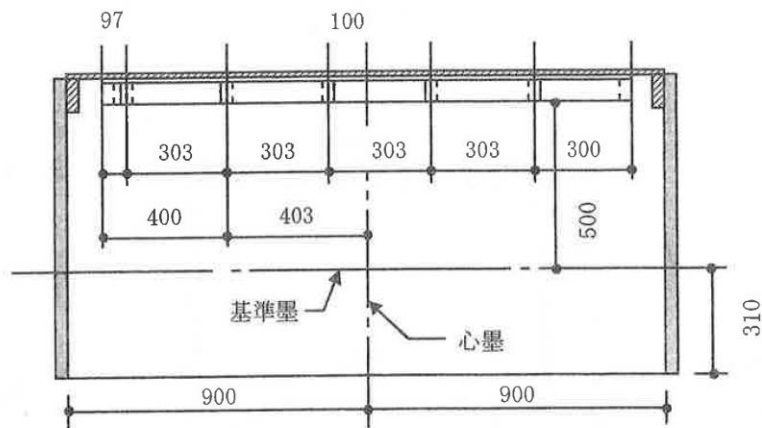
A-A 断面図
