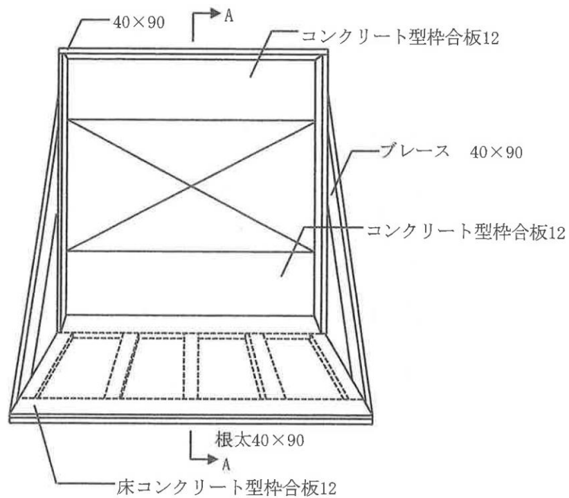
見 取 図
