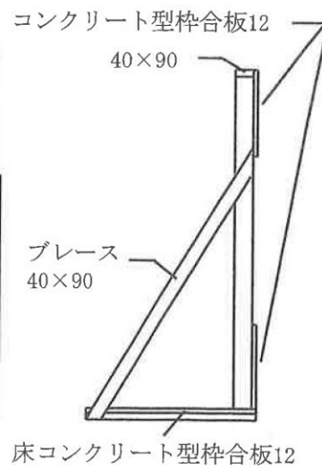
側面図
