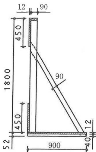
A-A断面図
