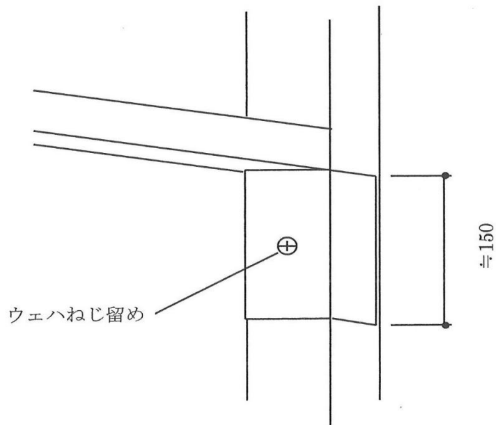
開口部ランナの固定方法
