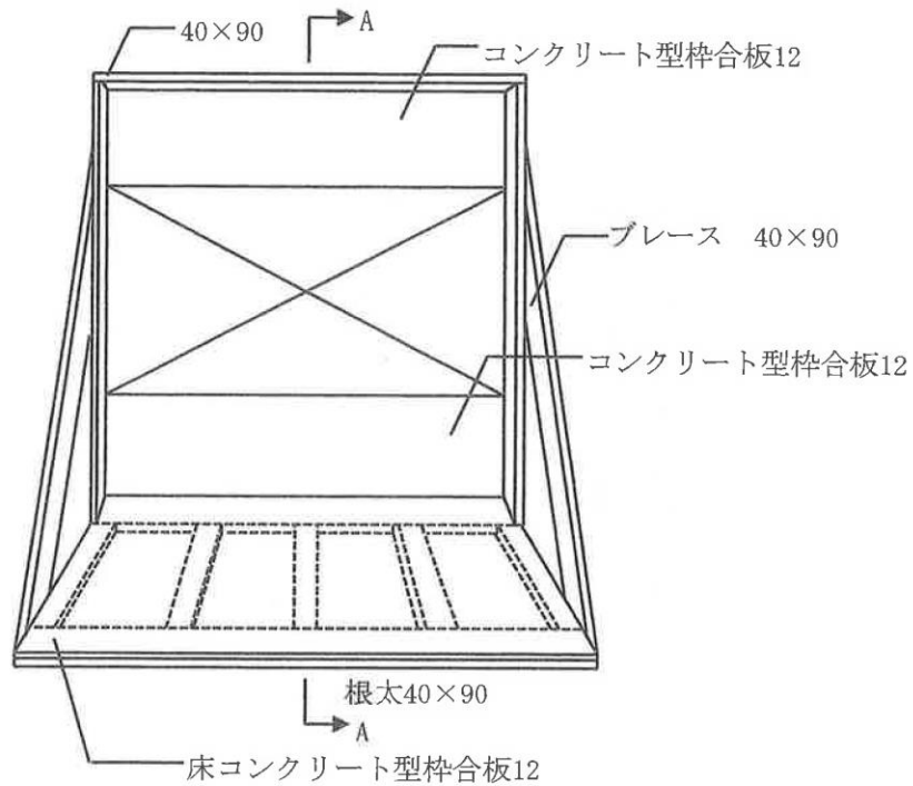
見取図
