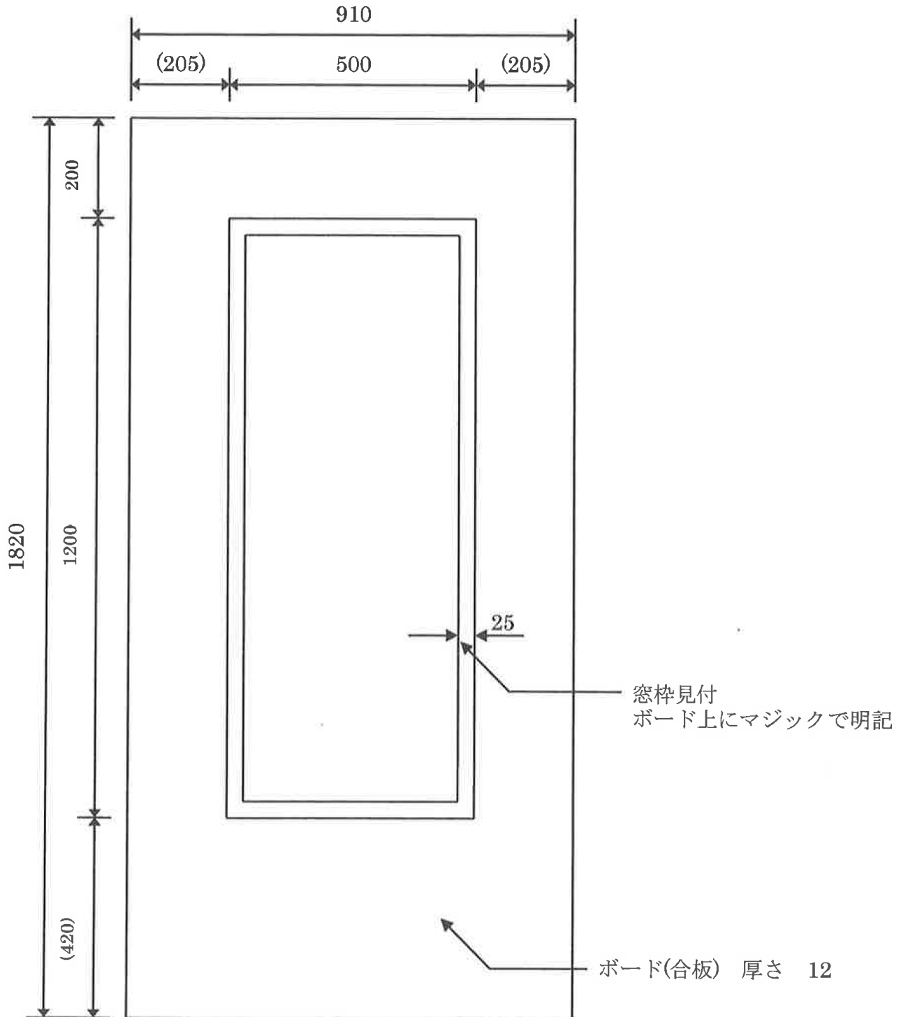
窓 枠 立 面 図
