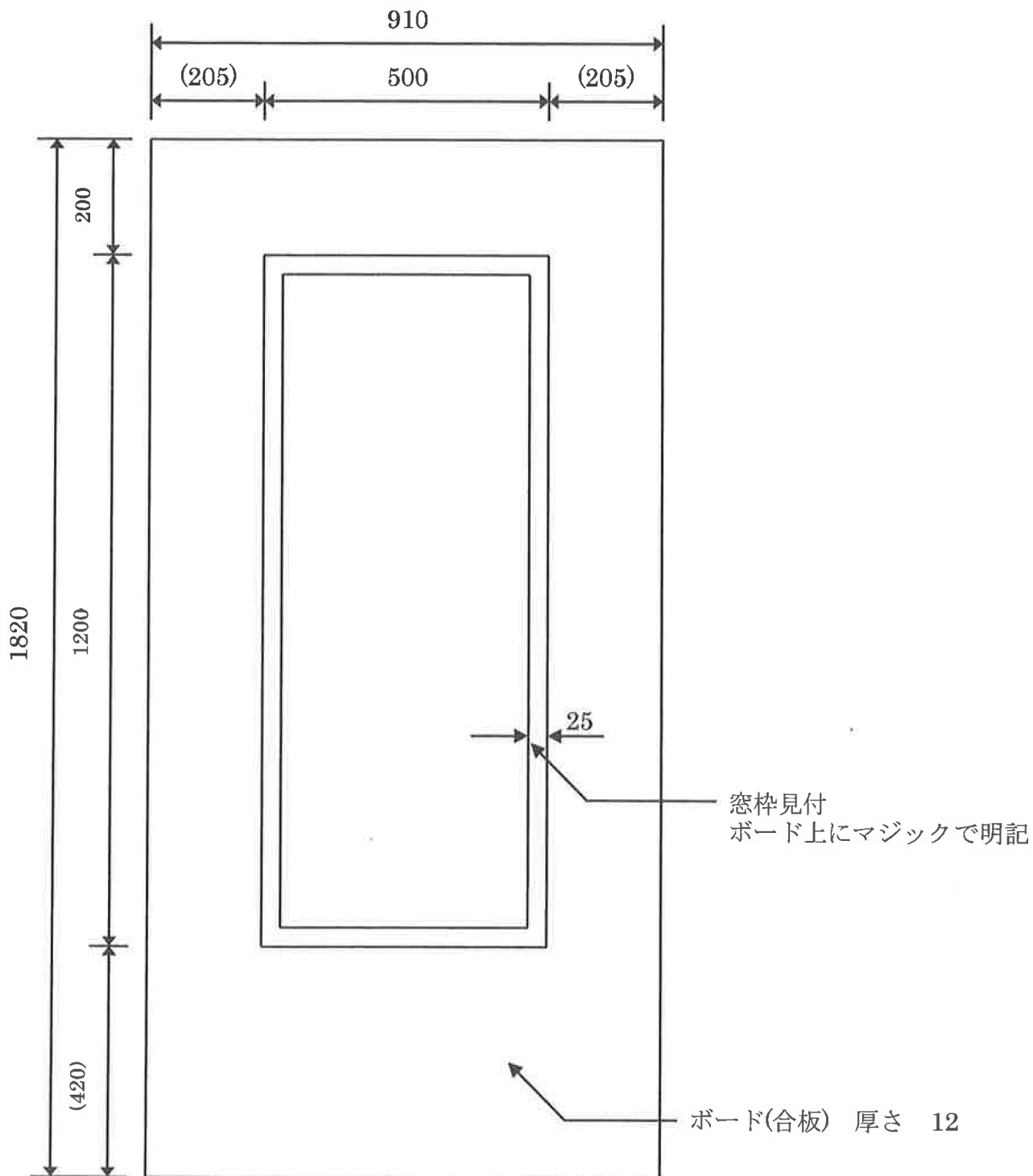
窓 枠 立 面 図
