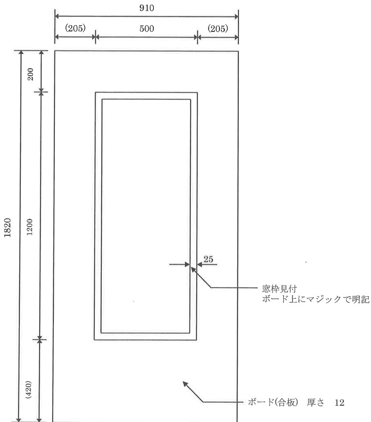
窓 枠 立 面 図
