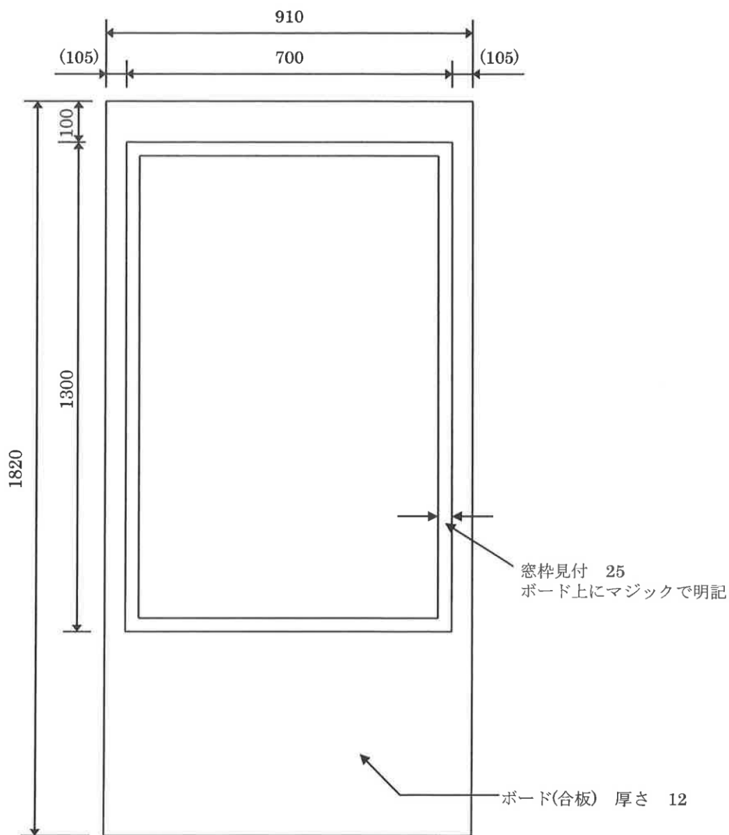
窓 枠 立 面 図
