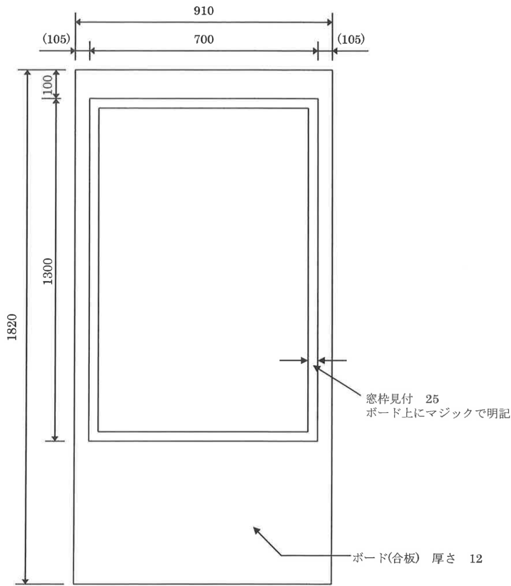
窓 枠 立 面 図
